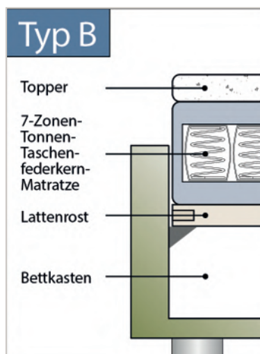
Typ B 7-Zonen-Tonnentaschenfederkern
