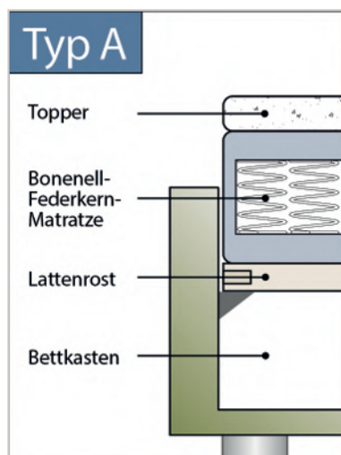
Typ A Bonnellfederkern
