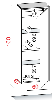
Re = Drehtür mit Rechtsanschlag
