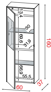
Li = Drehtür mit Linksanschlag
