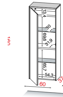
Li = Drehtür mit Linksanschlag
