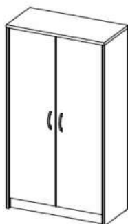
Art.Nr. 70-001-.. Hochschrank 2 Türen 4 E-Böden B/H/T ca. 72 x 148 x 35 cm Pal.-Menge 4
