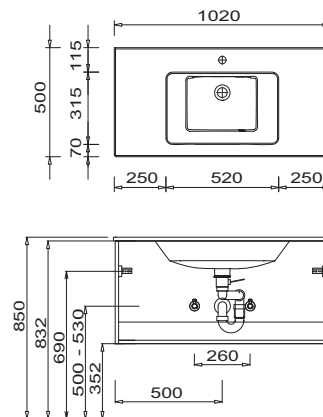
WTM 4410 1 Unterschrankhöhe 480 mm
