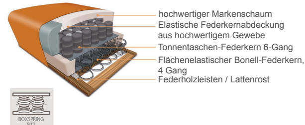
Boxspringsitz mit Bonell-Federkern und Tonnentaschenfederkern. Achtung! Bei dieser Ausführung erhöht sich die Sitzhöhe auf 48 cm!
