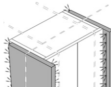
131 Seitenwangen M LED-Beleuchtung pro Wange – Lichtleiste vorne seitlich und hinten B 4,4 cm, T 63,6 cm
