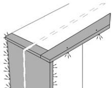
136 Seitenwange M LED-Beleuchtung pro Wange – Lichtleiste vorne seitlich und hinten und Kranz mit Spotbeleuchtung B 4,4, H 3,6, T 64,2 cm
