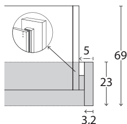
Draufsicht Schrank inkl. PPT-Rahmen
