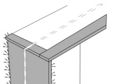
135 Seitenwange M LED-Beleuchtung pro Wange – Lichtleiste vorne seitlich und hinten und Kranz B 4,4, H 3,6, T 64,2 cm
