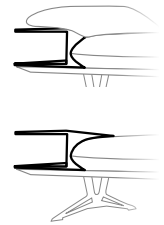
ARMLEHNE F ARMREST F Regal (optional mit Armteilkissen) Shelf (optionally with armrest cushion)
