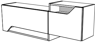
1x EA95-L, 1x EA52-R gesamt: 140 x 51 x 30 cm
