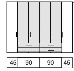
Breite = 269,2 cm
