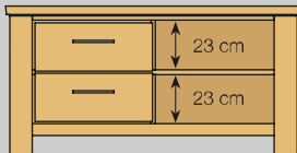
0204- Medienanrichte B 130 H 64 T 46 cm 2 Schubkästen, 2 offene Fächer lichtiges Maß der offenen Fächer: B 53 H 47 T 39 cm
