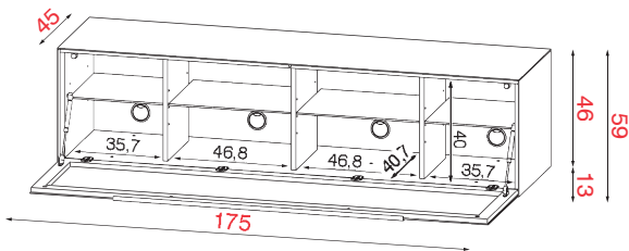
Korpushöhe 50 cm
