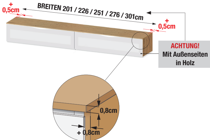
Holz-Abdeckplatte: Höhe 0,8cm
