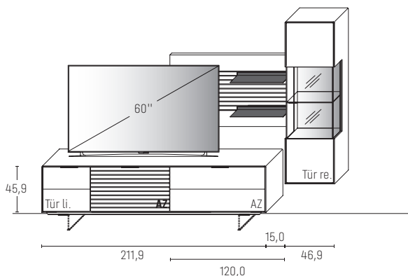
Fußgestell = Zubehör
