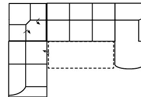
2BKL-ER-3FBB-OTTR Vorzugskombination
