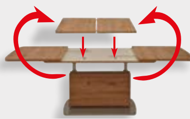
Synchro-Slice-Auszugsmechanik Beschreibung im Anhang
