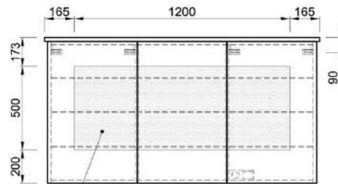
Optimaler Elektroanschlussbereich
