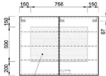
Optimaler Elektroanschlussbereich
