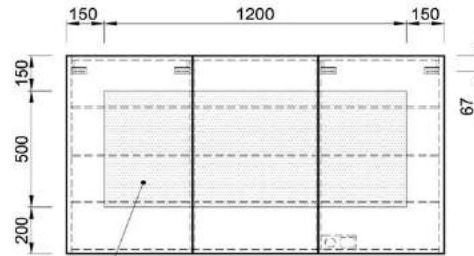
Optimaler Elektroanschlussbereich
