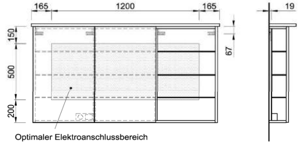
Spiegelschrank Typ 3 (Lichtkranzboden)
