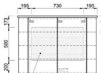
Optimaler Elektroanschlussbereich
