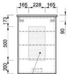
Optimaler Elektroanschlussbereich
