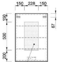
Optimaler Elektroanschlussbereich
