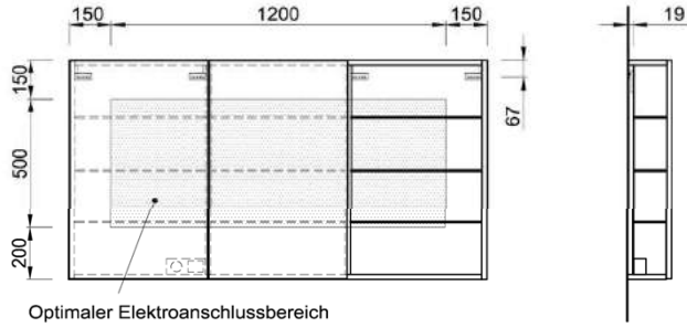
Spiegelschrank Typ 3 (Aufbauleuchte)
