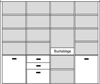
bestehend aus: Regalkorpus 12R 4 x 1272 Tür links 4R 1 x L_F044 Tür rechts 4R 1 x R_F044 Schubkastenpaar 1 x K024 Hoher Schubkasten 1 x K02H Buchablage 1 x 0171 PH 270_D
