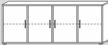
60368/40/F/G* 178x70x40cm (BxHxT) 60368/32/F/G* 178x70x32cm (BxHxT)
