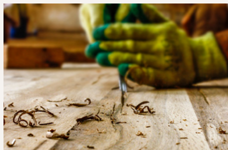
Ausarbeitung der Risse in Handarbeit mit Stechbeitel
