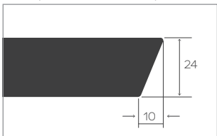
Kopfenden / Tabletop ends
