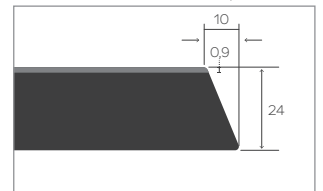
Tischseiten / Tabletop sites
