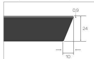
Kopfen / Tabletop ends
