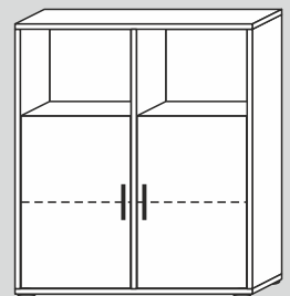
60164/40/F/G* 90x102x40cm (BxHxT) 60164/32/F/G* 90x102x32cm (BxHxT)
