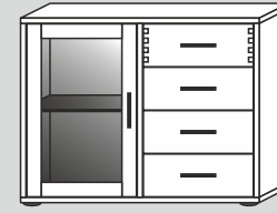
60114L/40/F/G* 90x70x40cm (BxHxT) 60114L/32/F/G* 90x70x32cm (BxHxT)
