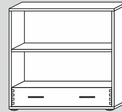
60119/40/F/G* 90x86x40cm (BxHxT) 60119/32/F/G* 90x86x32cm (BxHxT)
