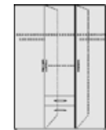
Drehtürenschränk 3-türig 2 Mittelwände 4 Einlegeböden 2 Kleiderstangen 2 Schubkästen
