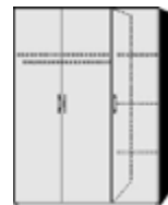
Drehtürenschränk 3-türig 1 Mittelwand 4 Einlegeböden 1 Kleiderstange
