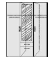
Drehtürenschränk 3-türig 1 kurze mittlere Tür mit Spiegel 2 Mittelwände 4 Einlegeböden 2 Kleiderstangen 2 Schubkästen
