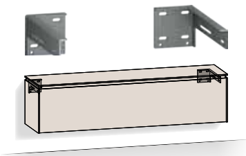
Optionale Beschläge für Wandmontage der Grundelemente
