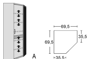
Eck-Element 1 Tür, rechts angeschlagen 1 fester Boden 4 verstellbare Böden Tür auf Wunsch auch links angeschlagen
