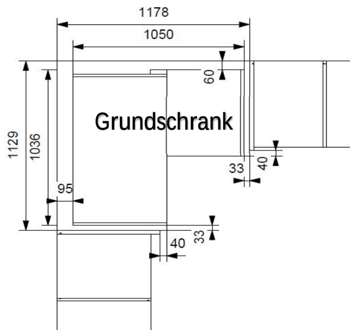
90° Ecke, 2-türig
