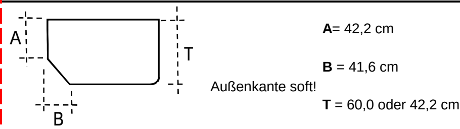
Detail Arbeitsplatte
