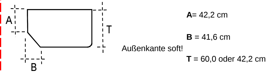
Detail Arbeitsplatte
