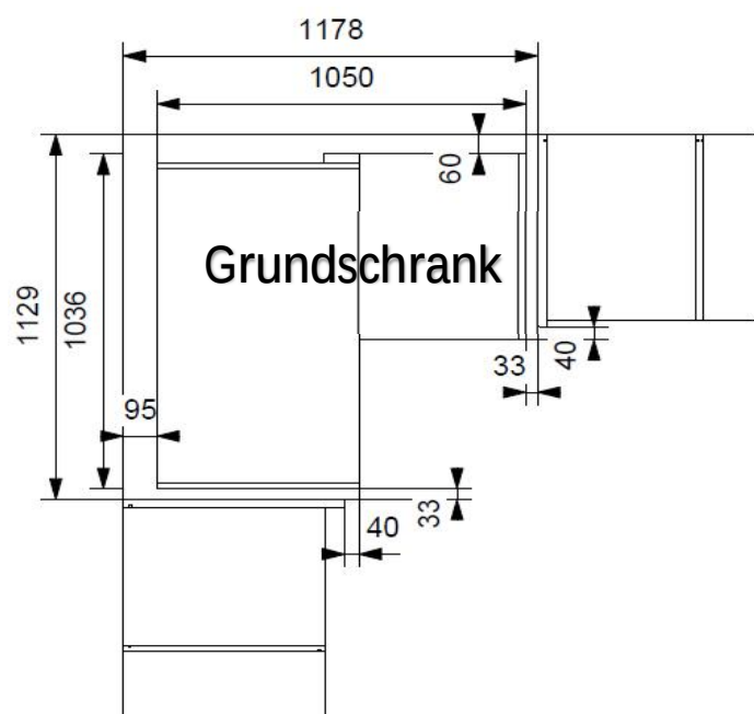
90° Ecke, 2-türig
