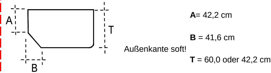
Detail Arbeitsplatte
