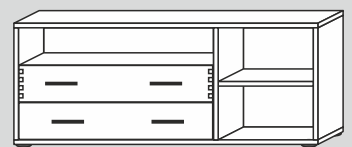
60214L/40/F/G* 134x54x40cm (BxHxT) 60214L/32/F/G* 134x54x32cm (BxHxT)
