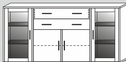
60392/40/F/G* 178x86x40cm (BxHxT) 60392/32/F/G* 178x86x32cm (BxHxT)
