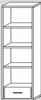
60517L/40/F/G* 46x134x40cm (BxHxT) 60517L/32/F/G* 46x134x32cm (BxHxT)
