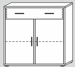
60134/40/F/G* 90x86x40cm (BxHxT) 60134/32/F/G* 90x86x32cm (BxHxT)
