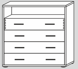
60124/40/F/G* 90x86x40cm (BxHxT) 60124/32/F/G* 90x86x32cm (BxHxT)
