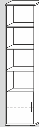
60715L/40/F/G* 46x182x40cm (BxHxT) 60715L/32/F/G* 46x182x32cm (BxHxT)
