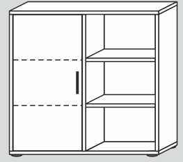
60129L/40/F/G* 90x86x40cm (BxHxT) 60129L/32/F/G* 90x86x32cm (BxHxT)
