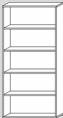
60723/40/F* 90x182x40cm (BxHxT) 60723/32/F* 90x182x32cm (BxHxT)
