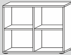
60102/40/F* 90x70x40cm (BxHxT) 60102/32/F* 90x70x32cm (BxHxT)
