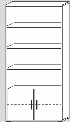
60740/40/F/G* 90x182x40cm (BxHxT) 60740/32/F/G* 90x182x32cm (BxHxT)
