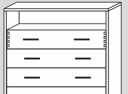
60124/40/F/G* 90x86x40cm (BxHxT) 60124/32/F/G* 90x86x32cm (BxHxT)
