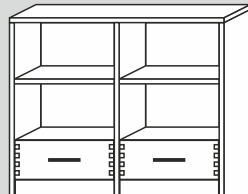
60122/40/F/G* 90x86x40cm (BxHxT) 60122/32/F/G* 90x86x32cm (BxHxT)
