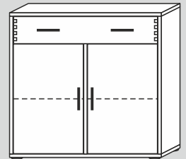
60134/40/F/G* 90x86x40cm (BxHxT) 60134/32/F/G* 90x86x32cm (BxHxT)
