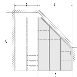
Dachschrägen-Anbauschränk 6044.10 .. 6210.10 .. B 46, H 224, T60 B 46, H 211, T60 Fertigung nur möglich mit Anbauschränk Art.-Nr. 6044.10.. oder 6210.10..
