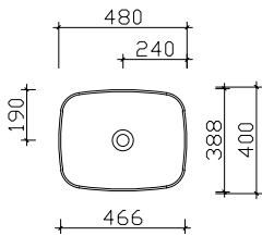
Breite 480 mm BAEN003M08010A
