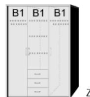
Drehtürenschränk 2 Mittelwände 5 Einlegeböden 2 kurze Kleiderstangen 3 Schubkästen
