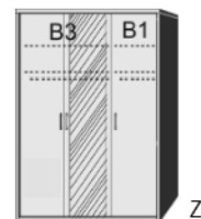
Drehtürenschränk 1 mittlere Tür mit Spiegel 1 Mittelwand 4 Einlegeböden 2 Kleiderstangen
