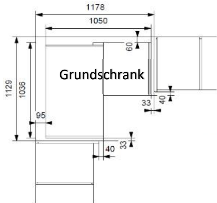
90° Ecke, 2-türig
