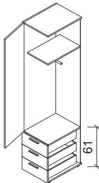
z Grundelement 1-türig mit 3 Schubkästen 45 cm
