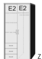
Drehtürenschränk 1 Mittelwand 4 Einlegeböden 1 kurze Kleiderstange 3 Schubkästen
