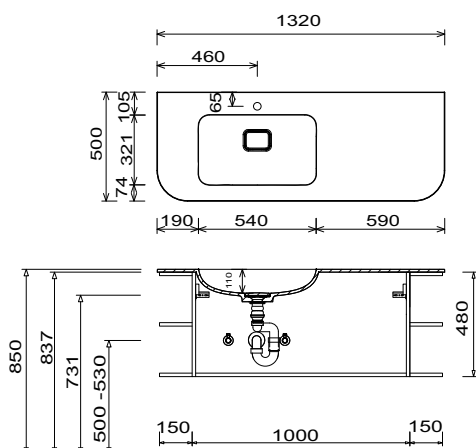
Beispiel Nizza rund Waschtisch Unterschrankhöhe 480 mm
