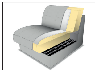
PUR-Schaum auf Wellenfedern (Standard)
