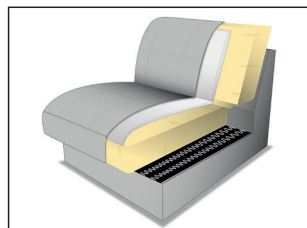
PUR-Schaum auf Wellenfedern (Standard)
