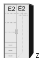
Drehtürenschränk 1 Mittelwand 4 Einlegeböden 1 kurze Kleiderstange 3 Schubkästen
