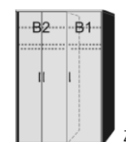
Drehtürenschränk 1 Mittelwand 4 Einlegeböden 2 Kleiderstangen
