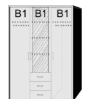
Drehtürenschränk 1 kurze mittlere Tür mit Spiegel 2 Mittelwände 5 Einlegeböden 2 kurze Kleiderstangen 3 Schubkästen
