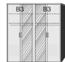
Drehtürenschränk 2 mittlere Türen mit Spiegel 1 Mittelwand 4 Einlegeböden 2 Kleiderstangen
