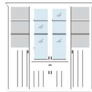
bestehend aus: Regalkorpus 12R 2 x 1249, 1 x 1295 Tür links 6R 1 x L_F062 Tür rechts 6R 1 x R_F062 Türenpaar mitte 3R mit Schubkasten mitte 1R 1 x FK47 Vitrinentürenpaar mitte 8R 1 x N087 H/G*
