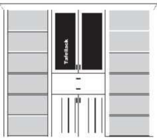
bestehend aus: Regalkorpus 12R 2 x 1272, 1 x 1295 Türenpaar 4R 1 x F047 Schubkastenpaar 2R 1 x K026 Türenpaar 6R (Tafellackfüllung) 1 x J067
