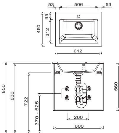
WSS 3660 41 + WUA 1260 G6 WSS 3660 41 + WUA 3360 G6
