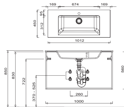
WSS 3610 41 + WUA 3310 G6
