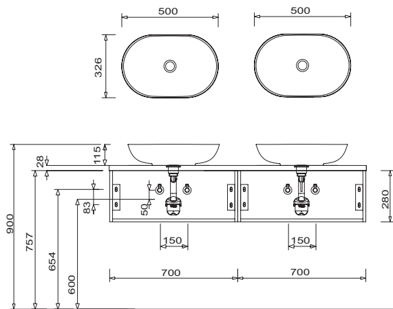
WSA 3250 41 + APA 4514 28 + WUA 124D G6 WSA 3250 41 + APA 4514 28 + WUA 334D G6
