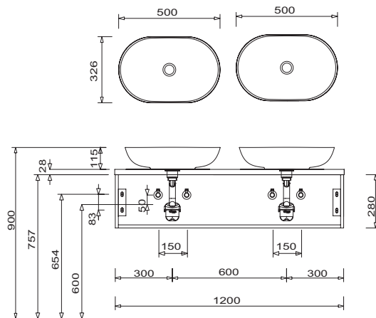
WSA 3250 41 + APA 4512 28 + WUA 12D2 G6
