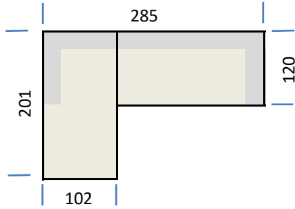
Type 001 - Longchair links, ohne Tiefenverstellung
