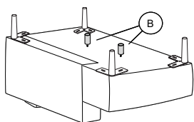
Umbauecke links/rechts
